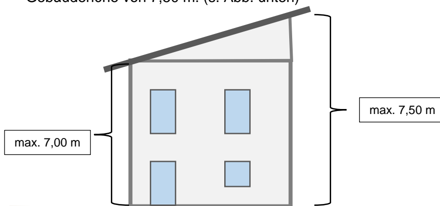
Abbildung: Gebäudehöhenregelung einhäufiges Pultdach ohne Staffelgeschoss | BBP
