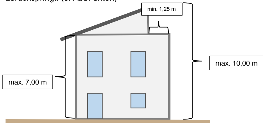
Abbildung: Gebäudehöhenregelung einhäufiges Pultdach mit Staffelgeschoss | BBP
